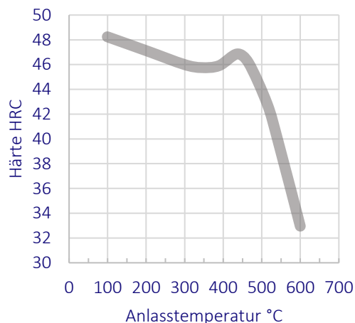
Anlassschaubild, Zustand: vergütet
