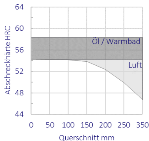
Härtbarkeit
