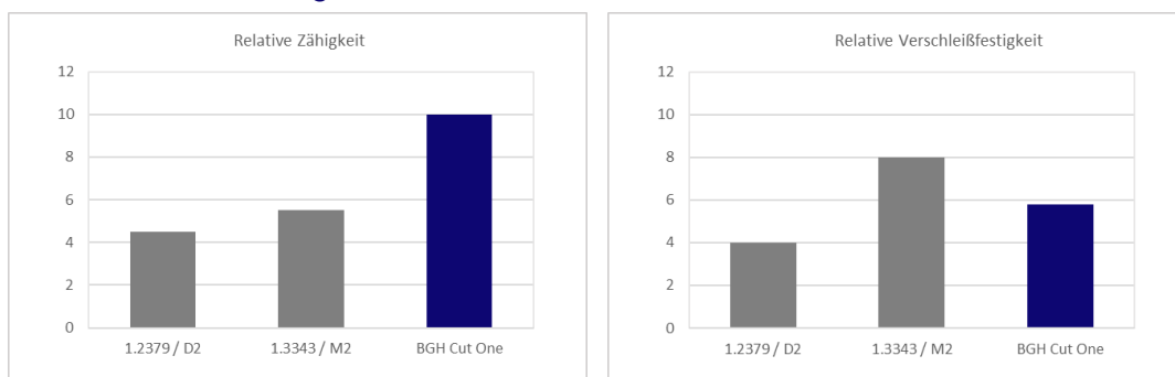
Abb. 1: Vergleich der Eigenschaften des BGH Cut One mit denen vergleichbarer Werkzeugstähle
